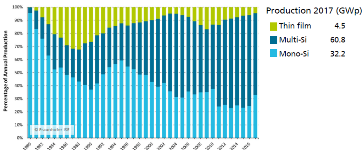
〈그림 5〉 박막·실리콘 태양광모듈 생산 추이
